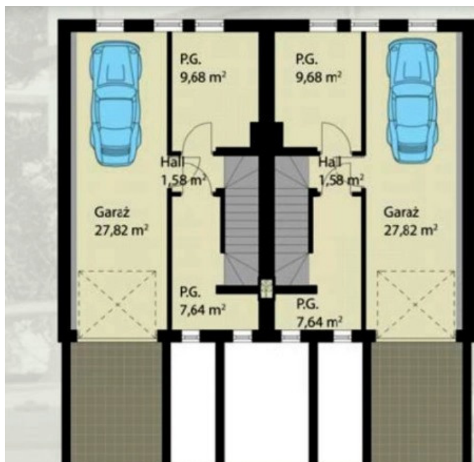
Rzut Przyziemia
